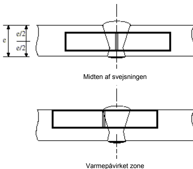
Varmepåvirket zone
