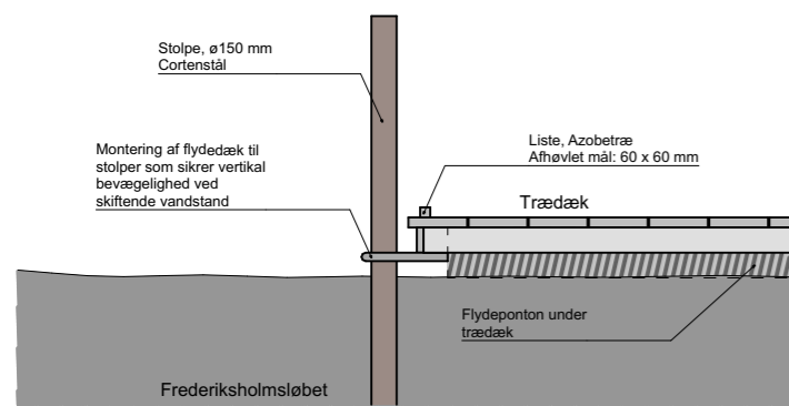
Principsnit, Flydeponten, 1:50
