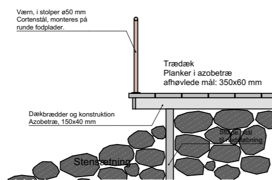
Principsnit, Trædæk og værn, 1:50
