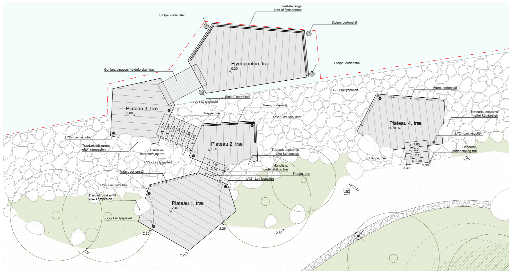
Planudsnit af trædæk, 1:100
