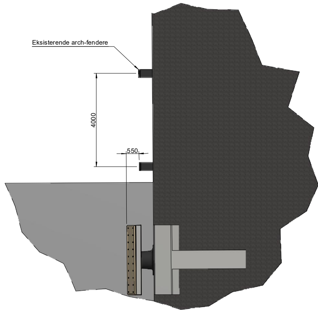
A ( 1 : 100 )
